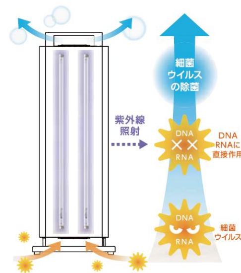
紫外線照射による除菌のしくみ
